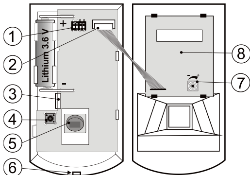
Obrázek 1: 1. DIP přepínač nastavení charakteristiky detektoru; 2. konektor; 3. západka; 4. sabotážní kontakt krytu; 5. PIR senzor; 6. západka krytu; 7. seřízení citlivosti MW; 8. mikrovlnný detektor
